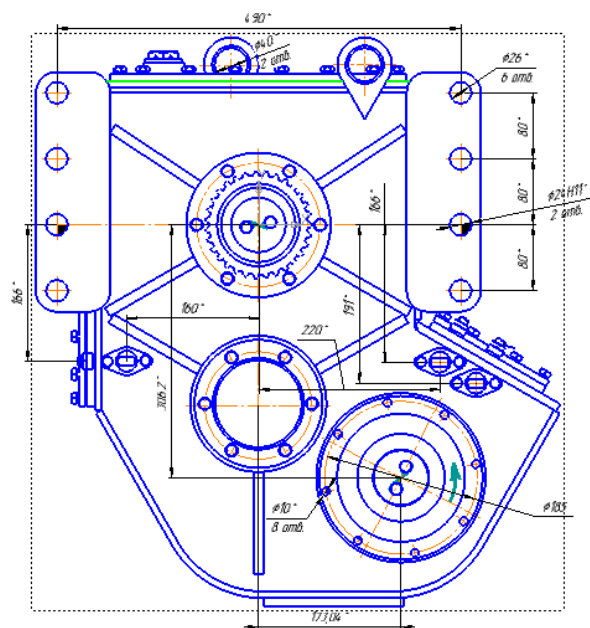
Рисунок 4 Вид сзади
