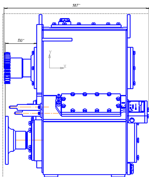
Рисунок 3 Вид сбоку
